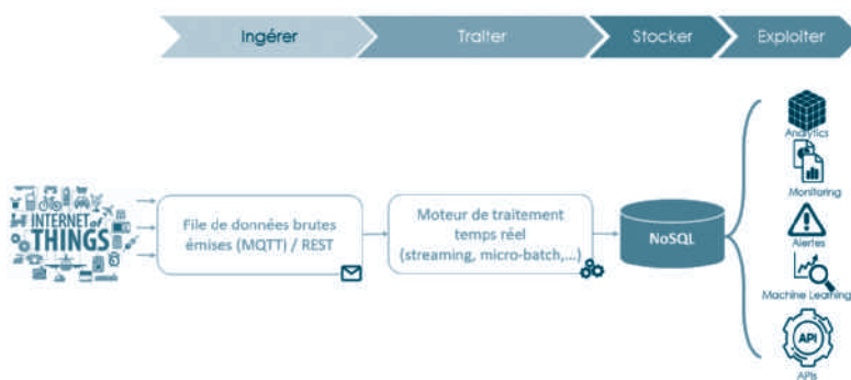
Modèle d'architecture générale de valorisation de données IIoT
